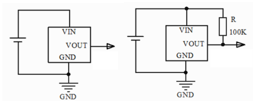
CMOS OUTPUT
